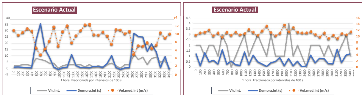
Parámetros medios globales. Alternativa 3. Izq, Sentido Decreciente. Dcha, Sentido Creciente. Av. de la Voluntat Popular. Elaboración propia
