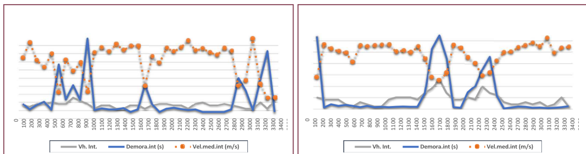
Parámetros medios globales. Alternativa 3 y 4. Izq, Sentido Decreciente. Dcha, SentidoCreciente. Av. de la Voluntat Popular.
