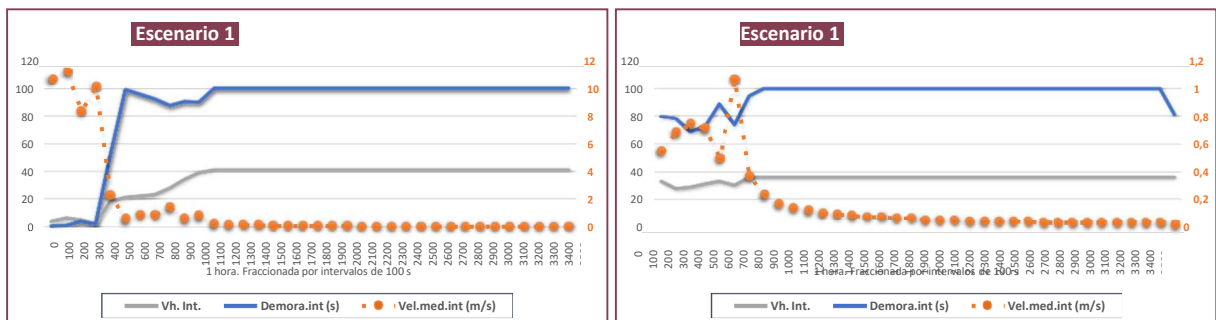
Parámetros medios globales. Alternativa 3. Izq, Sentido Decreciente. Dcha, SentidoCreciente. Av. de la Voluntat Popular.
