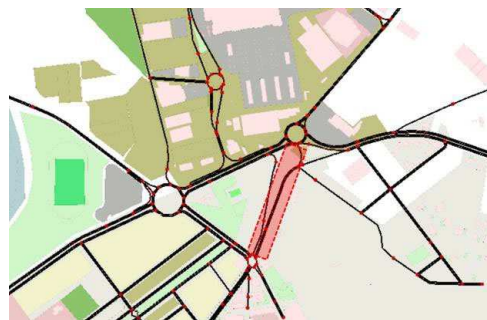
Alternativa 4-Glorieta Albalat introducida en el modelo de tráfico.
