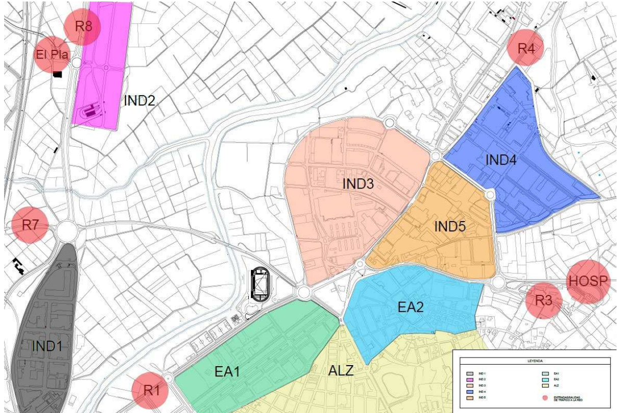
Disgregación de la red modelizada en zonas generadoras y atractoras de tráfico.
