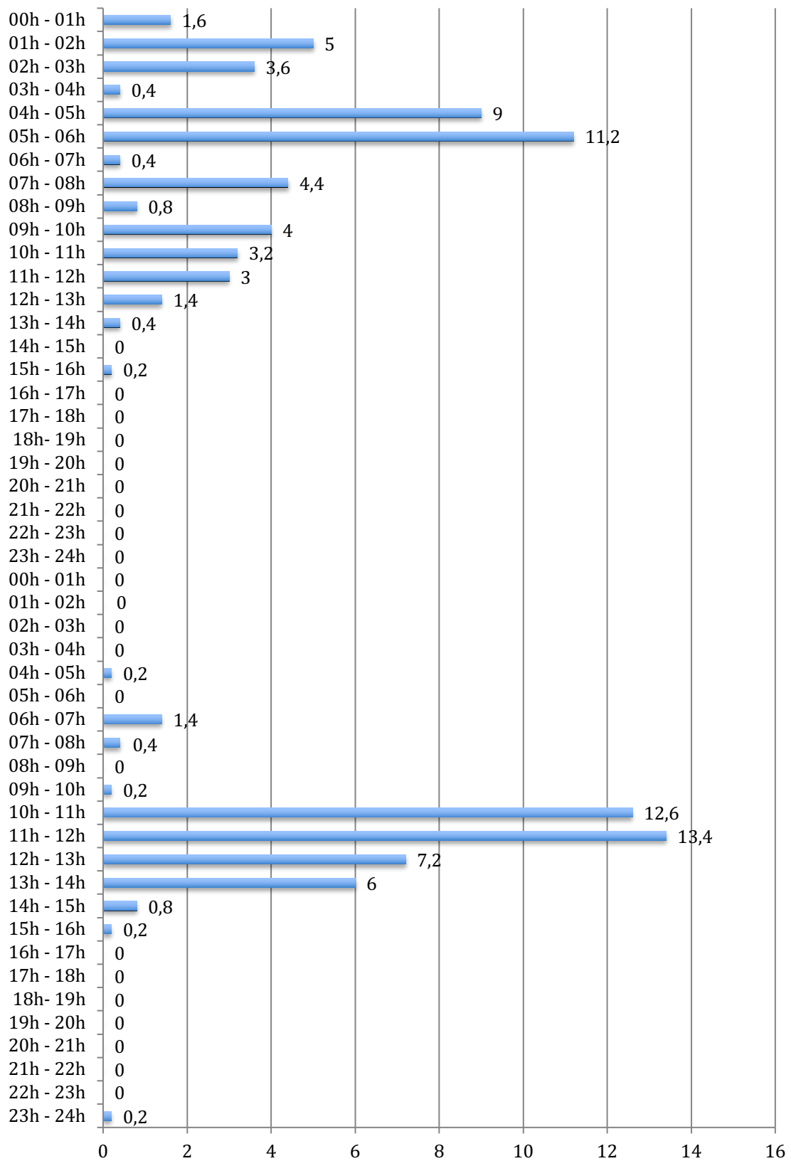
Cantidades de lluvia registradas por horas en ALZIRA los días 21 y 22/01/20 (en l/m 2 )
