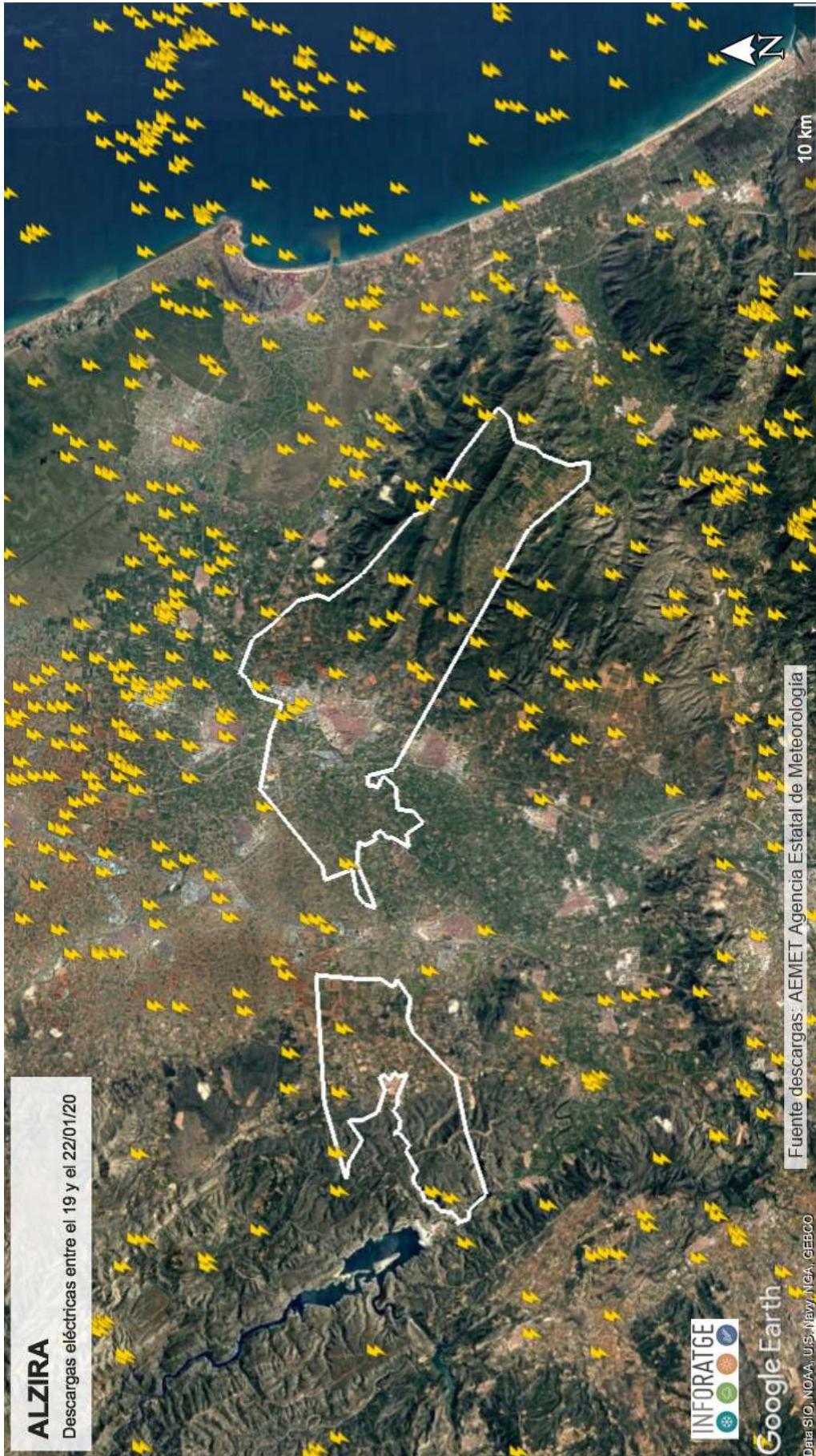
Geolocalización de las descargas eléctricas ~ nube-tierra registradas en el término municipal de ALZIRA y alrededores entre el 19 y el 22/01/20 Fuente descargas: AEMET Agencia Estatal de Meteorología
